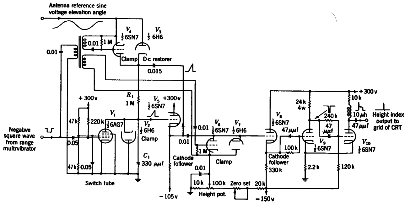
FIG. 6-18.—Height-index circuit.
