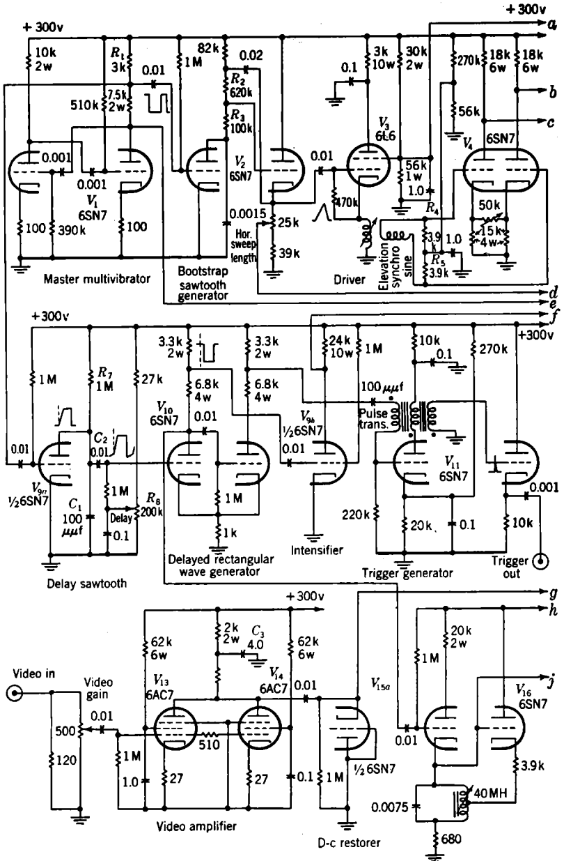
FIG. 15-6.—Range-height
