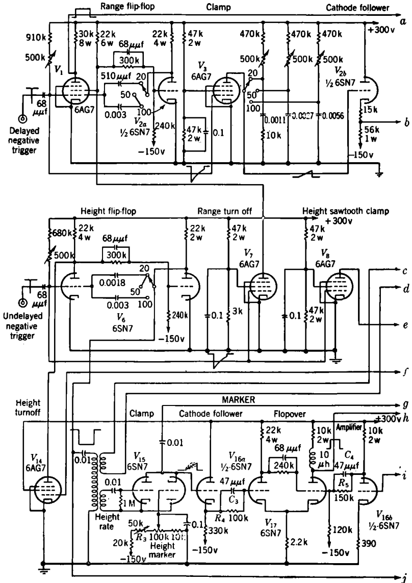
FIG. 15-7.—Range-height
