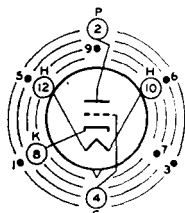
12AQ INDEX = LARGE LUG ● = SHORT PIN - IC
